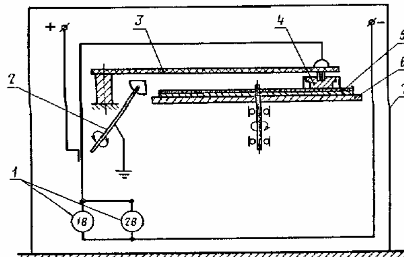
1 - киловольтметры; 2 - заземленный поворотный рычаг; 3 - подвижный рычаг; 4 - головка; 5 - кассета с образцом; 6 - диск; 7 - камера
